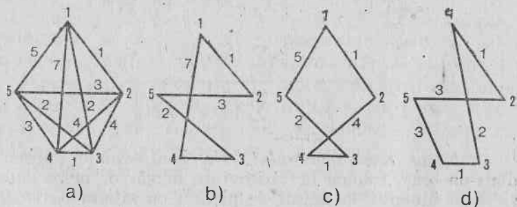
Fig. 8.1. Problema comis-voiajorului
