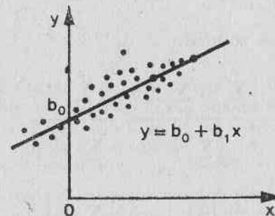
Fig. 3.19. Regresie liniară
