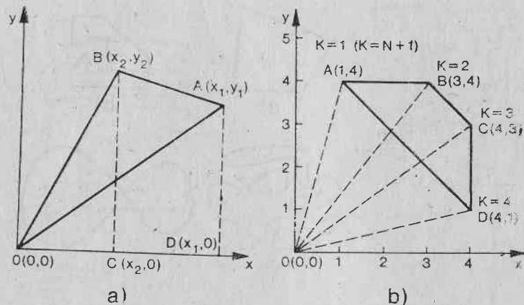
Fig. 3.4. Calculul ariei pe baza triunghiului
