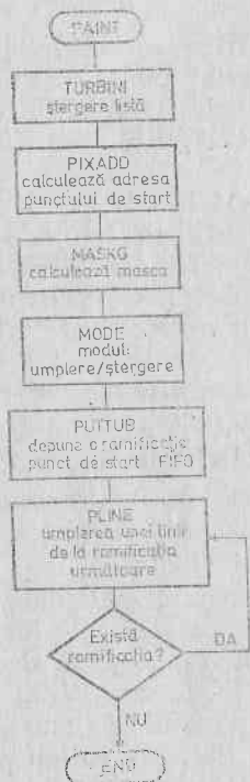
Fig. 5.5. Schema logică a rutinei PAINT
