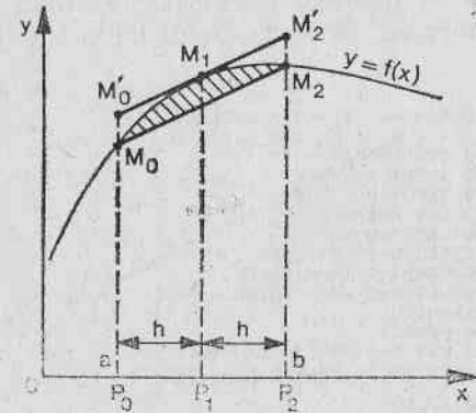
Fig. 3.17. Reprezentarea funcției
