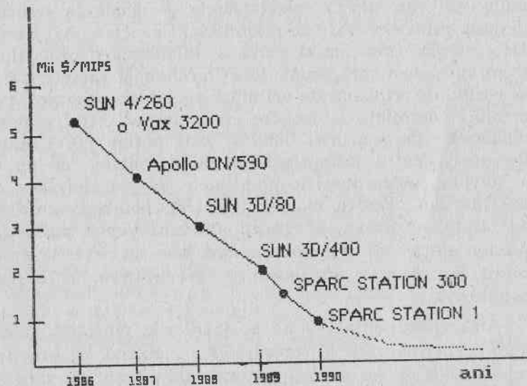
Fig. 9.2. Raportul cost/performanță
