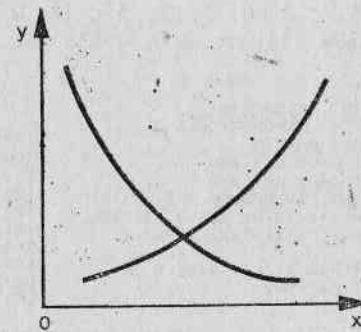
Fig. 3.24. Funcția exponențială y = ab^x
