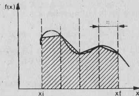
Fig. 3.7. Metoda trapezelor
